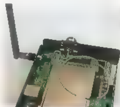
D-Link DWL-900AP+ geopend met N-chassisdeel in plaats van interne antenne.
